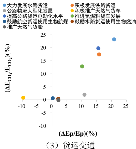
图 4-1 市内客运关键措施的 CO 2 与空气污染物综合当量减排协同效应
