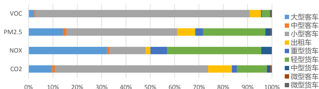
(a) 广州大道北分车型的排放分担率
