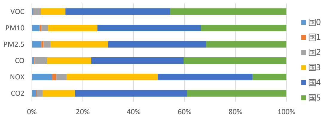
(a) 广州大道北不同排放标准车型的排放分担率
